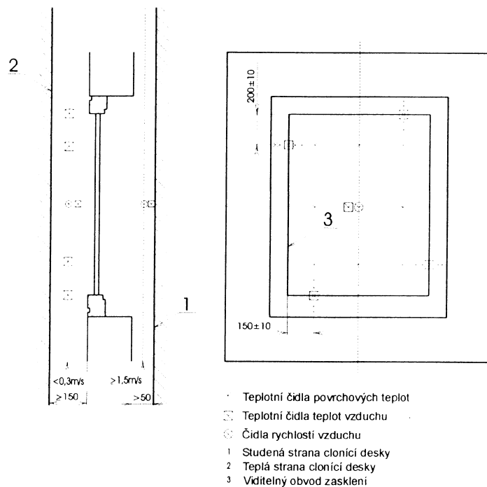
Obrázek 4 Rozmístění teplotních a rychlostních čidel na výřezu okenního profilu
